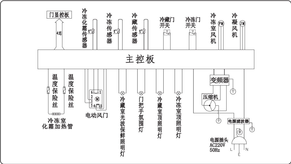
电路图（BCD-593WD02GBIWS）
