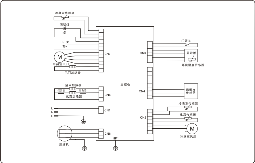
电路图（BCD-432WMGBWS）
