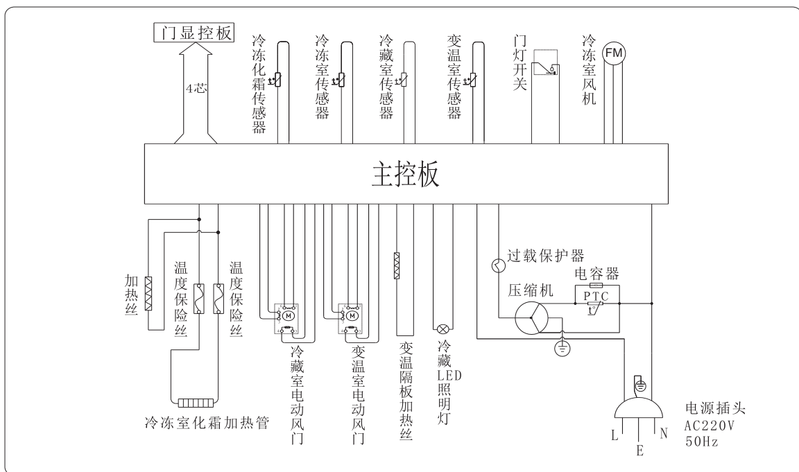
电路图 (BCD-263WTGEW/BCD-263WT07GWS)
