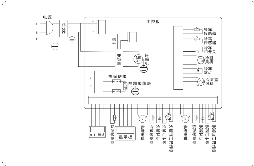
电路图 (BCD-576WDGBIWS)
