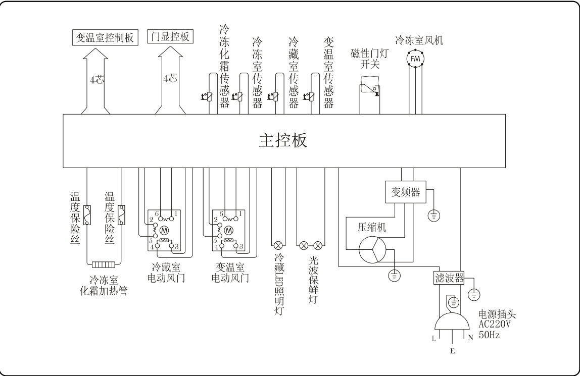
电路图（BCD-343WTGBW）
