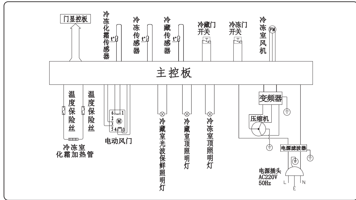
电路图 (BCD-593WDGBFW)
